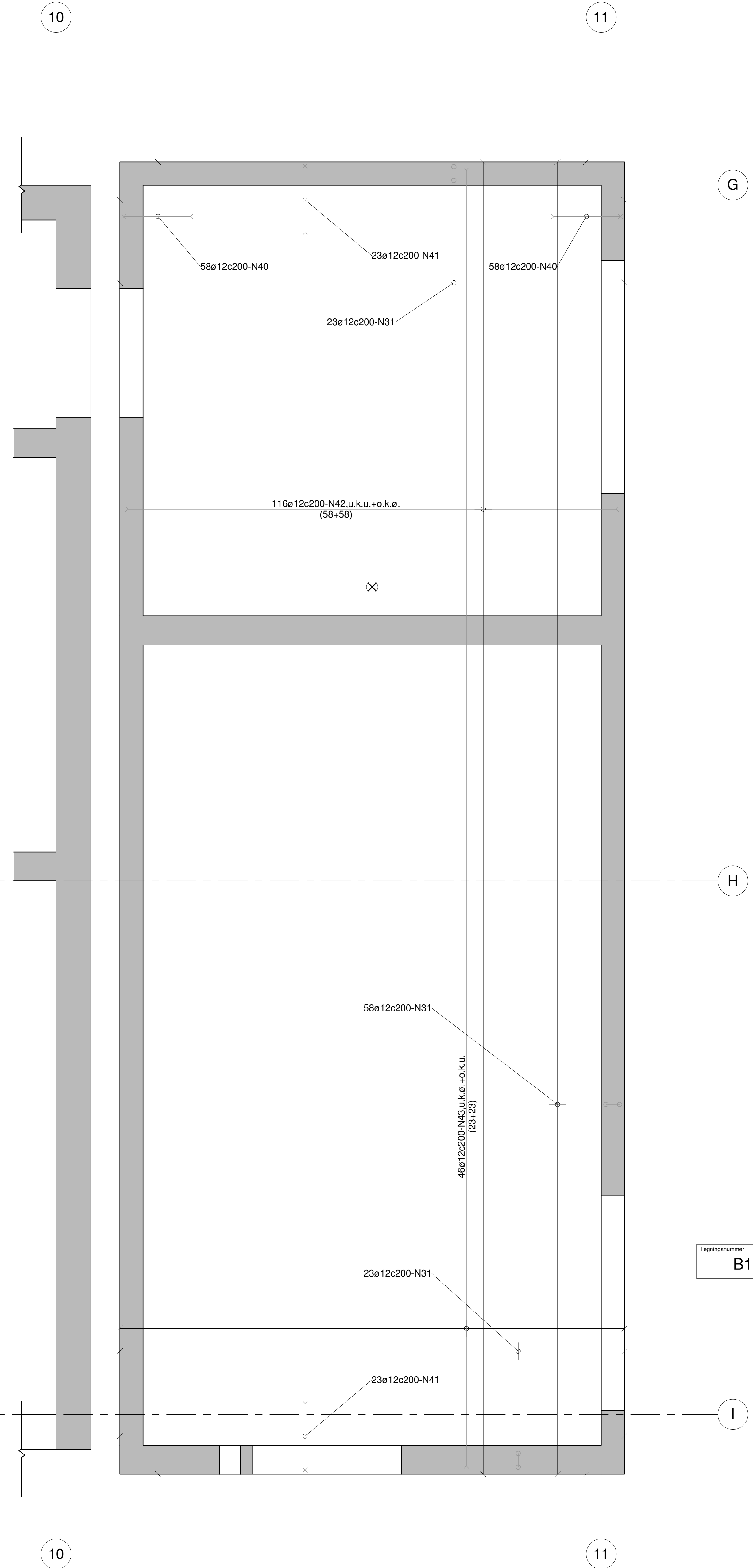
DEKKE OVER TRAFØ 1:20
